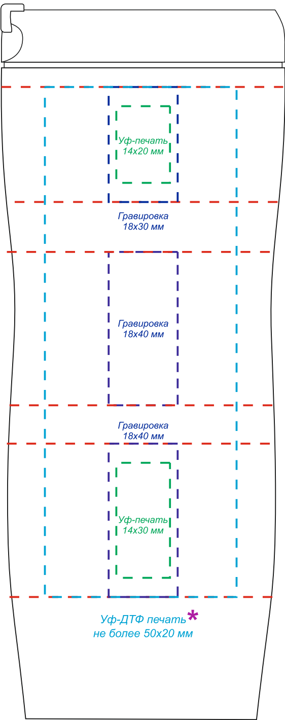
Вид справа
