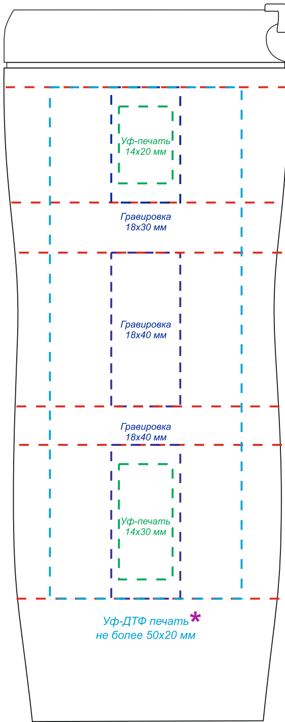
Вид слева
