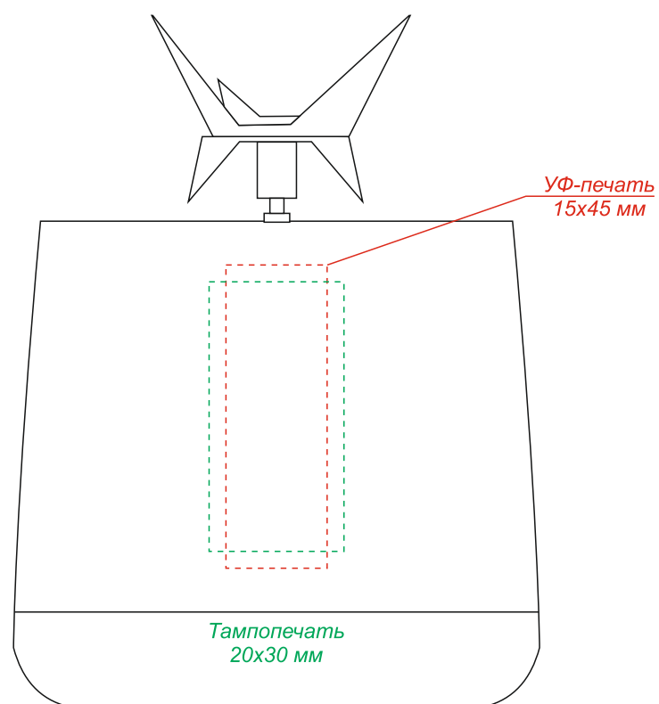
Вид сбоку (справа, слева)
