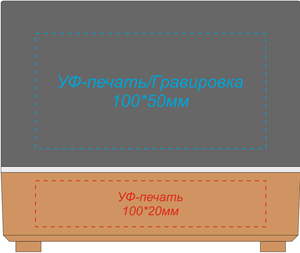
Вид сзади
