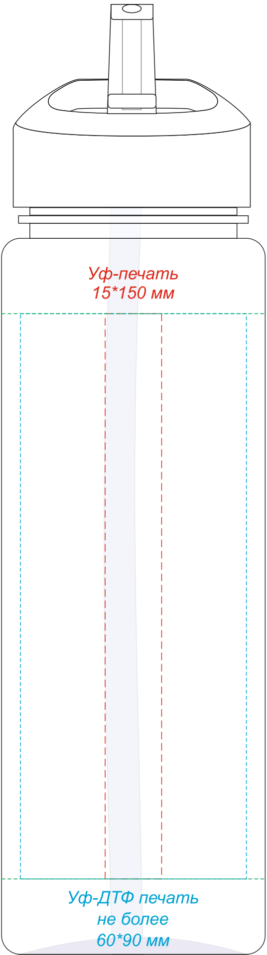
вид спереди
