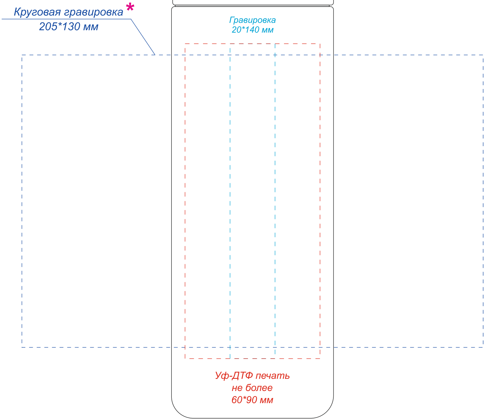
вид спереди
