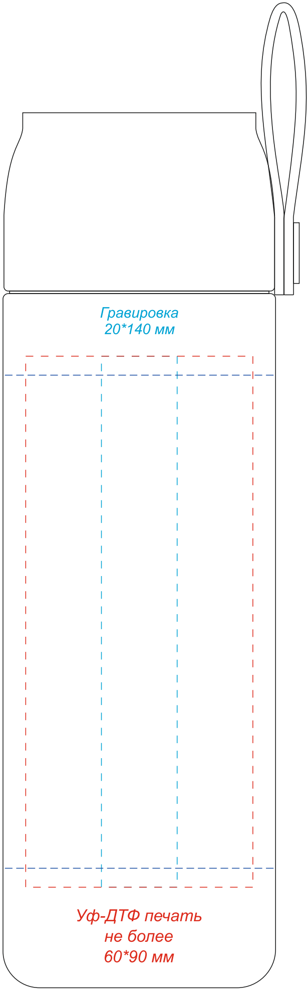
вид справа
