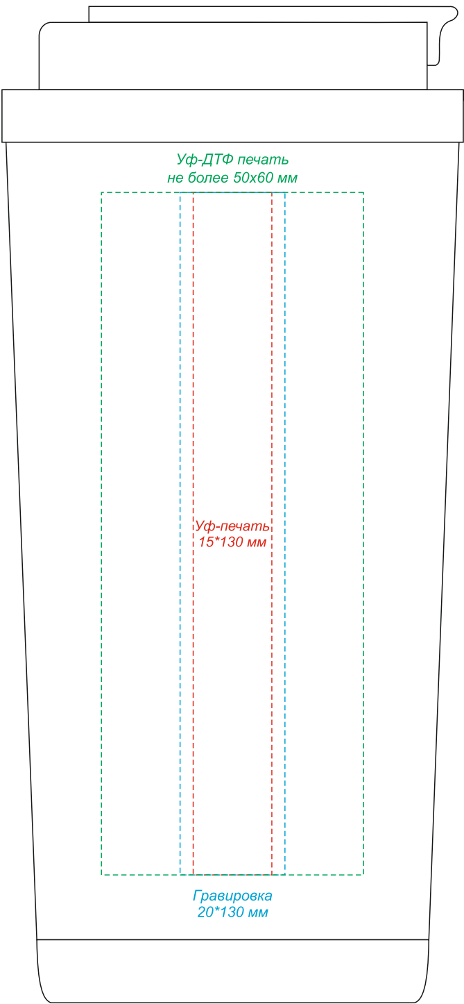
вид слева
